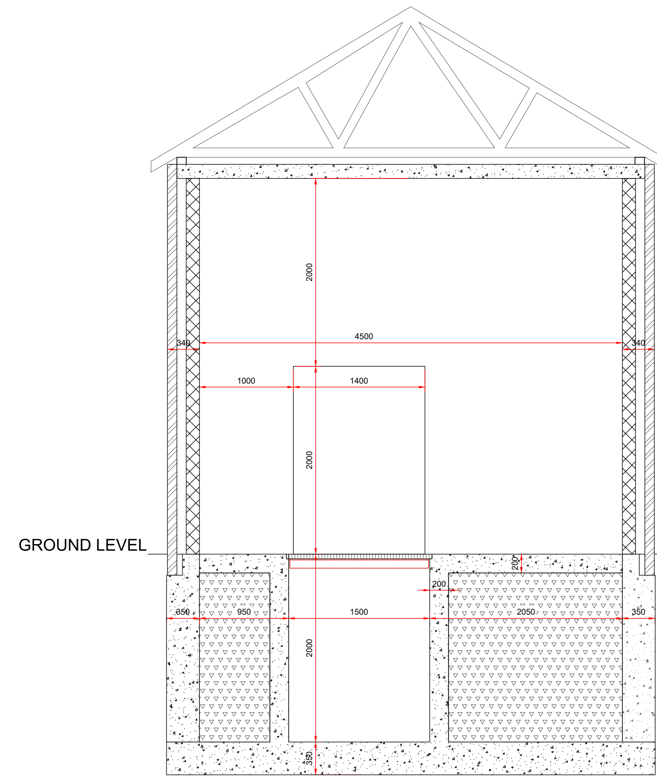
SECTION D-D
