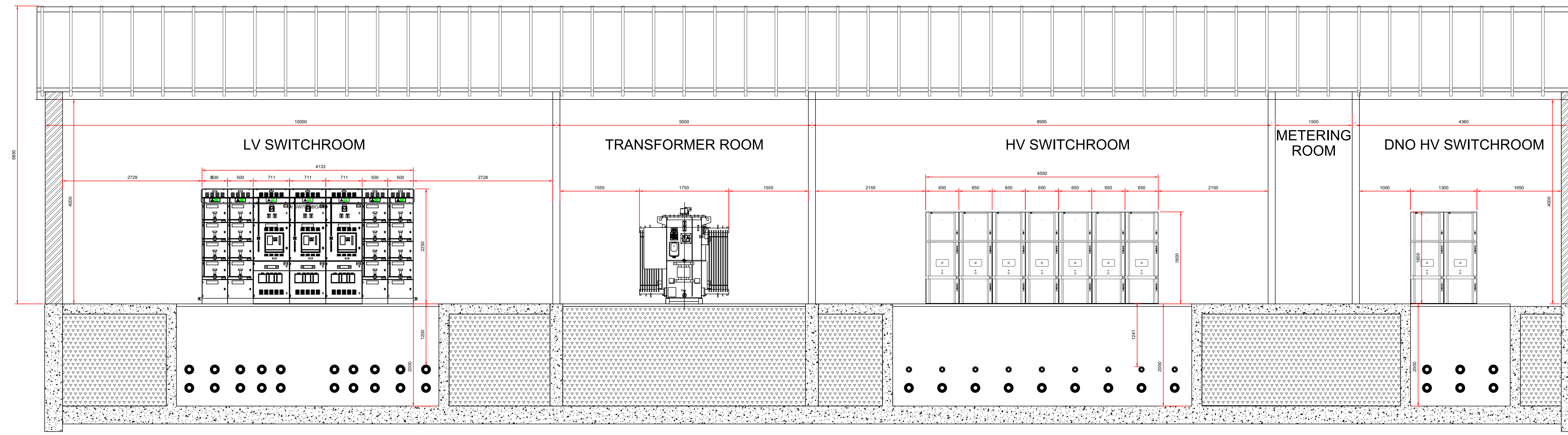
SECTION A-A
