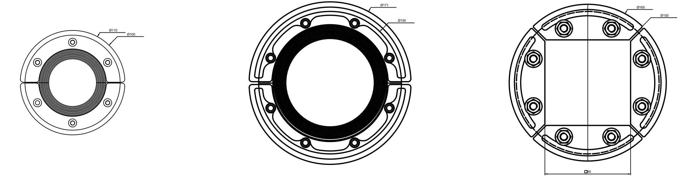
DETAIL A: 100mm RS ROXTEC UNIT
